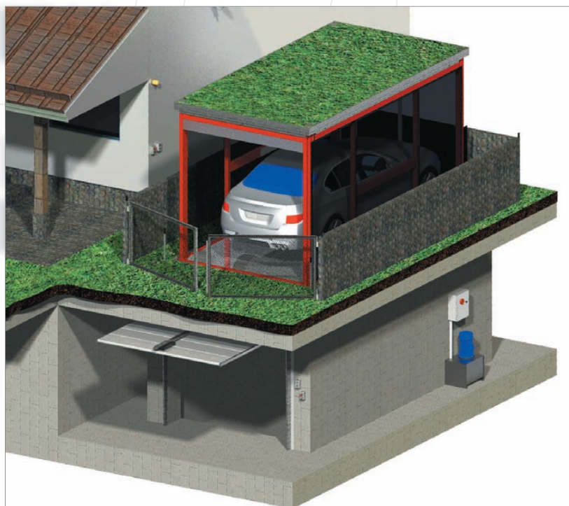
Esempio di applicazione con Sistema SPB (richieste protezioni perimetrali)
